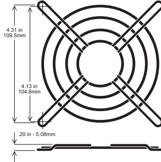
MFG120-W8-LF
