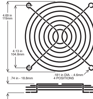
MFG120-W3-LF
