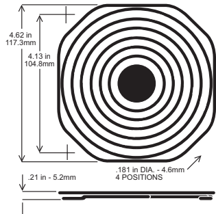
MFG120-W6-LF
