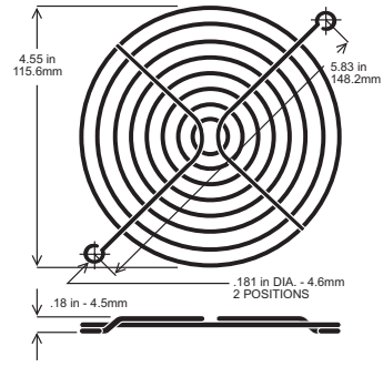
MFG120-W10-LF
