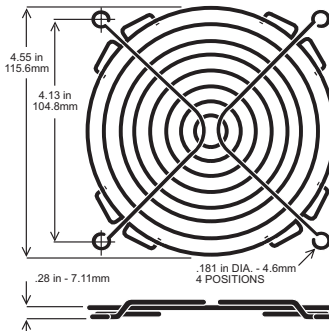
MFG120-W15-LF
