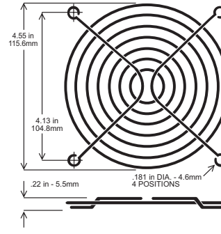
MFG120-W4-LF
