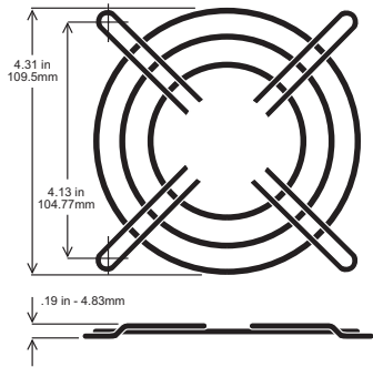
MFG120-W14-LF
