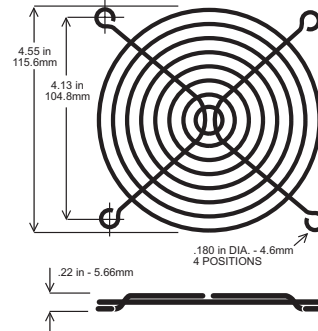
MFG120-W16-LF
