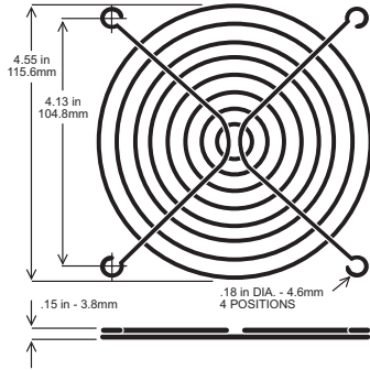
MFG120-W2-LF
